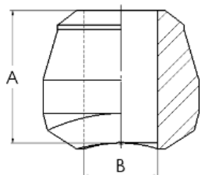
B.W. end Extrémité Butt-welding
