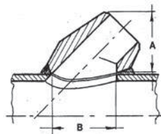
B.W. end Extrémité Butt-welding
