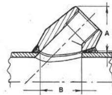
Threaded end Extrémité filetée
