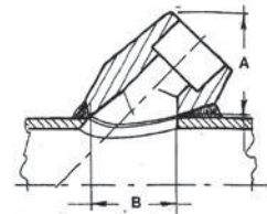
Socket-weld end Extrémité à souder
