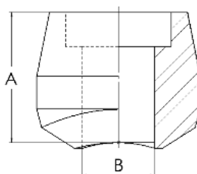
Socket-weld end Extrémité à souder
